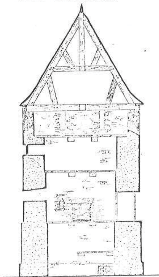
Duursdoorsnede van de "Tomp"
