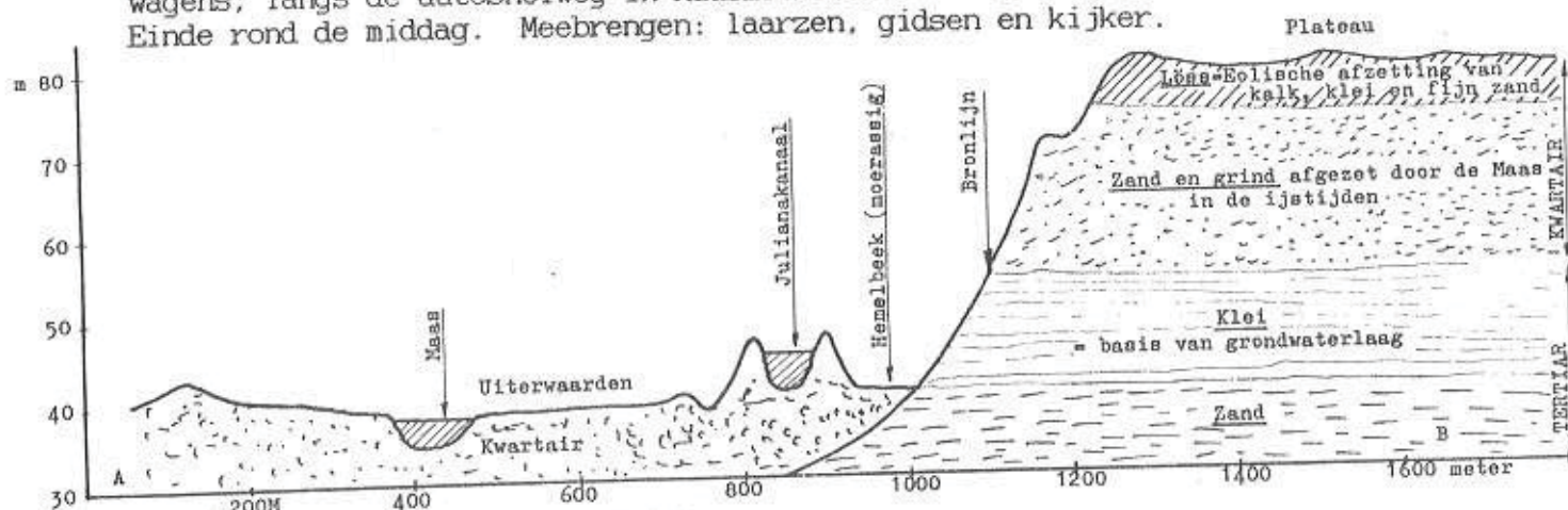
West - Oost profiel door het Bunderbos bij Elsloo Lengteschaal: 1/6666 Hoogteverdringing : 10X
