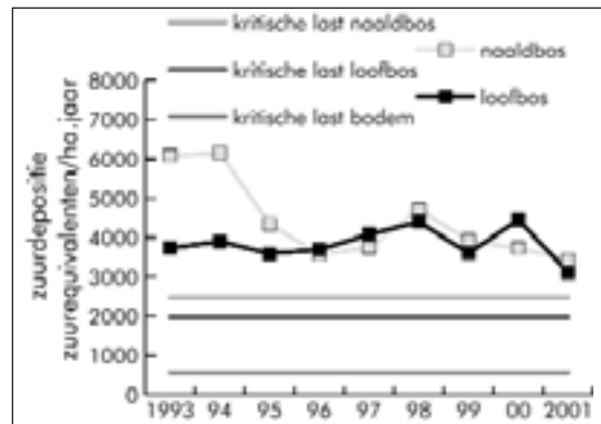
Evolutie van de zuurneerslag op 5 meetpunten van de intensieve opvolging van bossen (Wijnendale, Gontrode, Zoniën, Brasschaat en Ravels), in vergelijking met enkele kritische lasten. (Bron: De Schrijver A. et al., 2002).
