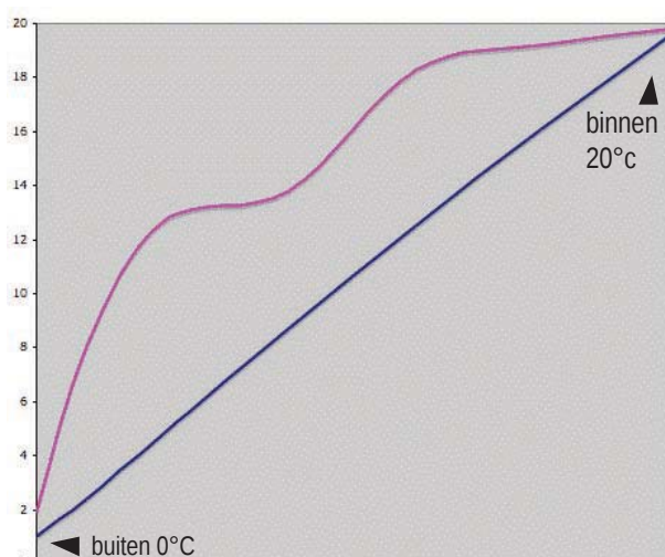
Temperatuurverloop in een muur van 20 cm dik
