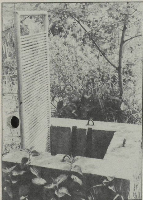
Het waterniveau-regelingsapparaat (=monnik), onmisbaar middel voor de regeling van de waterstand zonder onsnapping van vissen.
