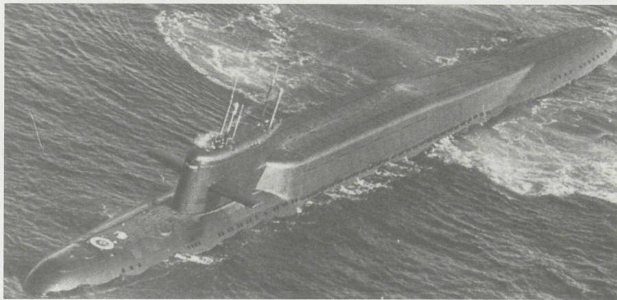
De Delta-duikboot was één van de paradepaardjes van de 'Noordelijke Vloot'. Dit type atoomduikboot was 160 meter lang, werd aangedreven door 2 kernreactoren en had 16 SS-N-8-kernraketten aan boord.
